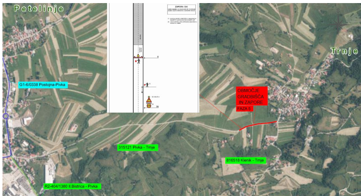
Slika 3: Prikaz območja popolne zapore ceste z oznako LC 315121 Pivka – Trnje (povzeto iz projektne dokumentacije, ki jo je podjetje PIZ Projektiva in inženiring Zasavje d.o.o. izdelalo marca 2025)
