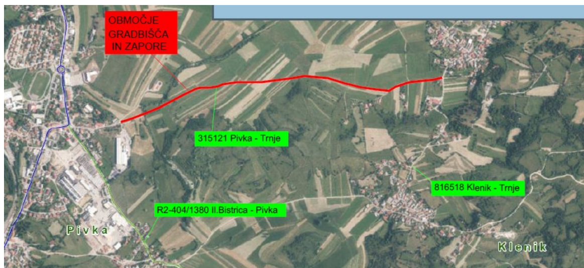
Slika 1: Pregledna situacija območja gradbišča in zapore ceste z oznako LC 315121 Pivka – Trnje (povzeto iz projektne dokumentacije, ki jo je podjetje PIZ Projektiva in inženiring Zasavje d.o.o. izdelalo marca 2025)
